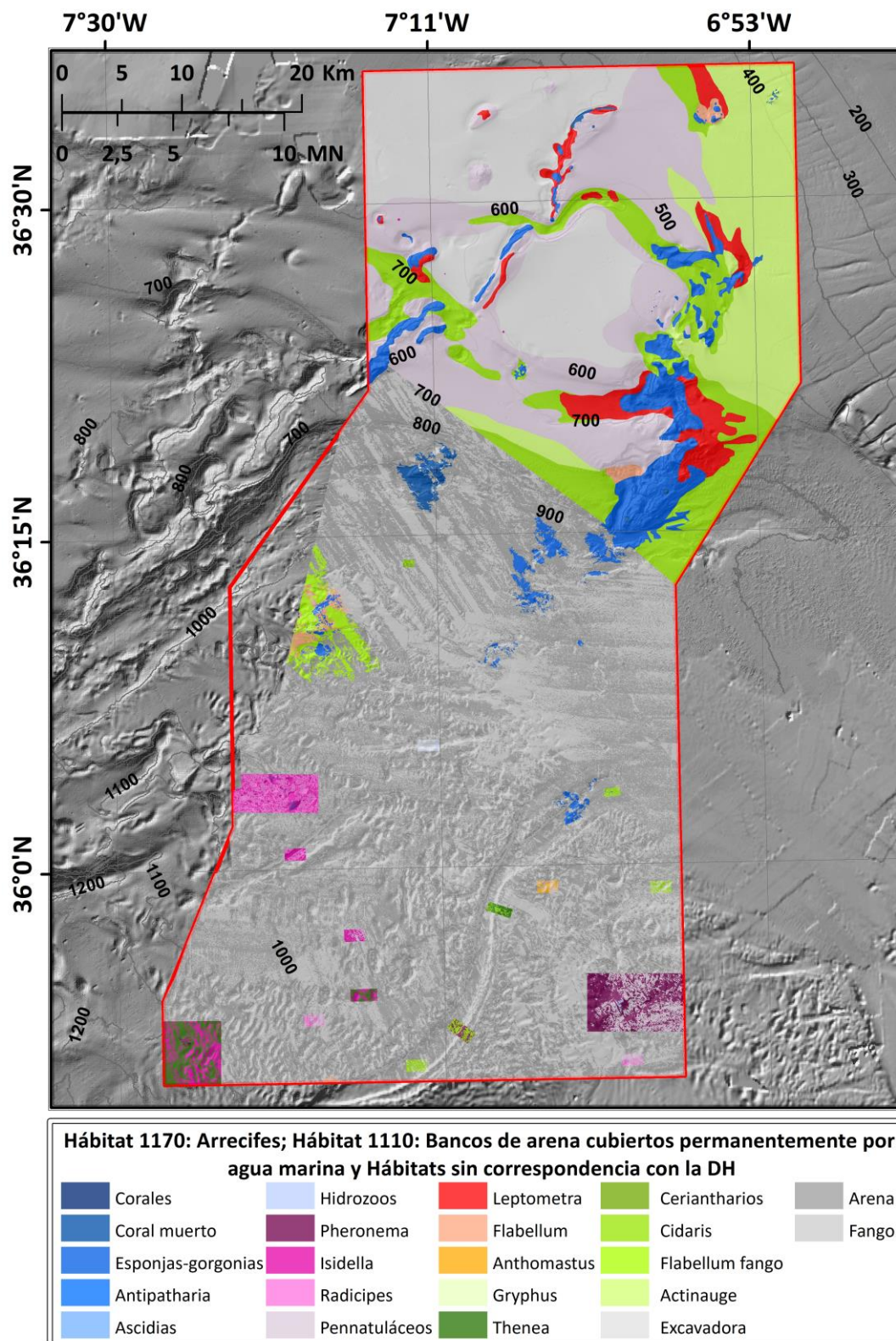
Figura 4. Distribución de los hábitats 1170, 1110 y los que no tienen correspondencia con directivas ni convenios en el LIC " Volcanes de fango del golfo de Cádiz ". En ANEXO de Rueda et al. (2022 b) se adjuntan mapas a mayor resolución del Campo Somero y Campo Profundo de Expulsión de Fluidos del LIC.
