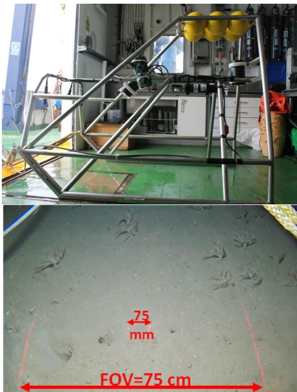
Figura 30. Detalle del trineo fotogramétrico HORUS y de los punteros láseres puntuales (separados 75 mm) y los lineales (separados 75 cm) en un fotograma submarino tomado con dicho trineo.
