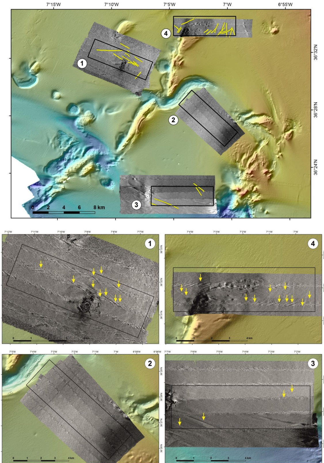
Figura 50. Polígonos en los que se han observado marcas de arrastre (cartografiadas con líneas amarillas arriba y marcadas con flechas amarilla abajo) a partir de datos de reflectividad de la ecosonda multihaz (mosaicos en escala de gris) obtenidos durante la campaña INTEMARES A4 CAD.
