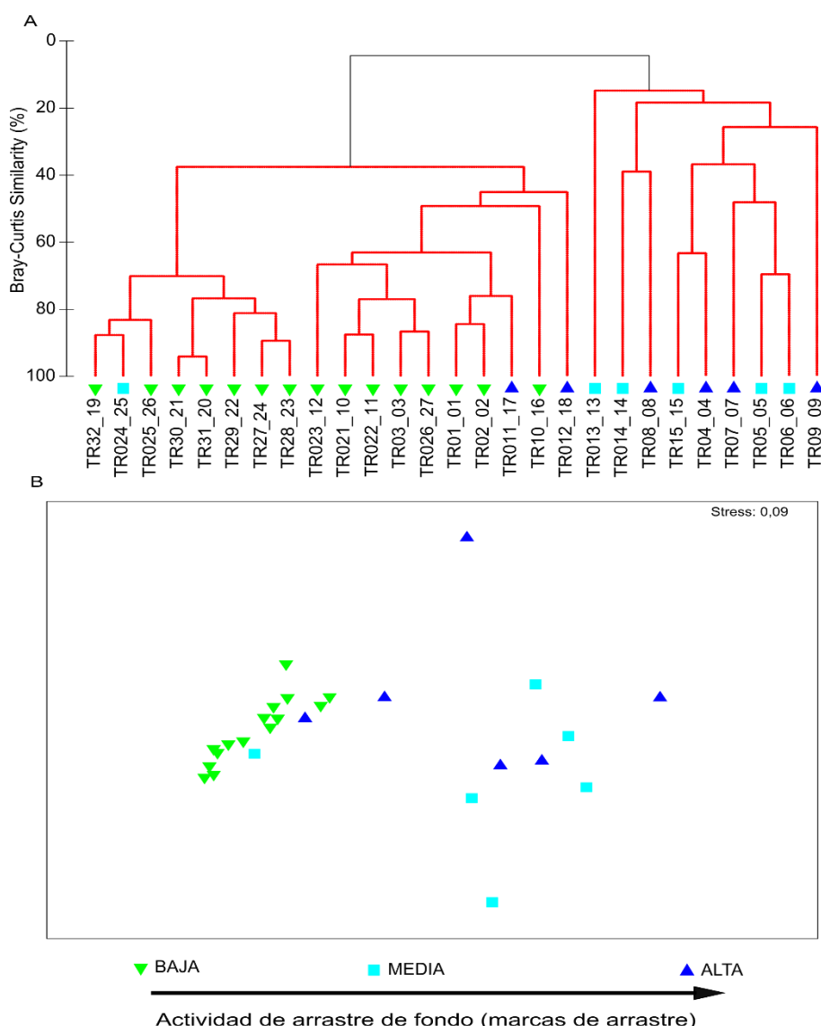
Figura 66. Cluster y nMDS basado en el índice de Bray-Curtis de los datos de abundancia (sin transformar) de las imágenes submarinas en relación al factor Marcas arrastre. Líneas rojas muestras agrupaciones significativas en base al test de SIMPROF ( p < 0,01 ).
