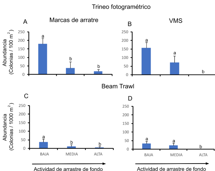
Figura 74. Abundancia media y error estándar del pennatuláceo Kophobelemnion stelliferum en transectos de imágenes submarinas (izquierda) y muestras de beam-trawl (derecha) con relación a los factores (A) de marcas de arrastre y (B) y horas de arrastre (SSB -VMS).
