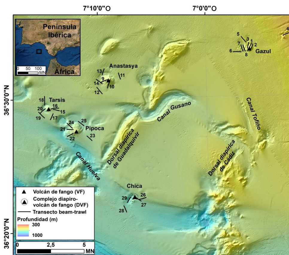
Figura 24. Localización de lances de beam-trawl en los diferentes sectores del Campo Somero de Expulsión de Fluidos del margen español del golfo de Cádiz durante las campañas INDEMARES-CHICA 0610 y CHICA 0211. Sectores: Gazul, Anastasya, Tarsis, Pipoca y Chica. Las coordenadas de los lances de beam-trawl se muestran en González-García et al. (2020b).
