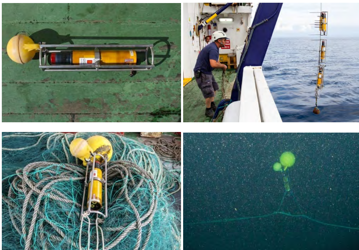
Foto 7. Baliza de Posicionamiento Acústico HIPAP (arriba y derecha); prueba de carga y transmisión de las balizas usadas en el experimento (arriba e izquierda); baliza amarrada al aparejo (abajo e izquierda); y baliza transmitiendo debajo del agua (abajo y derecha).
