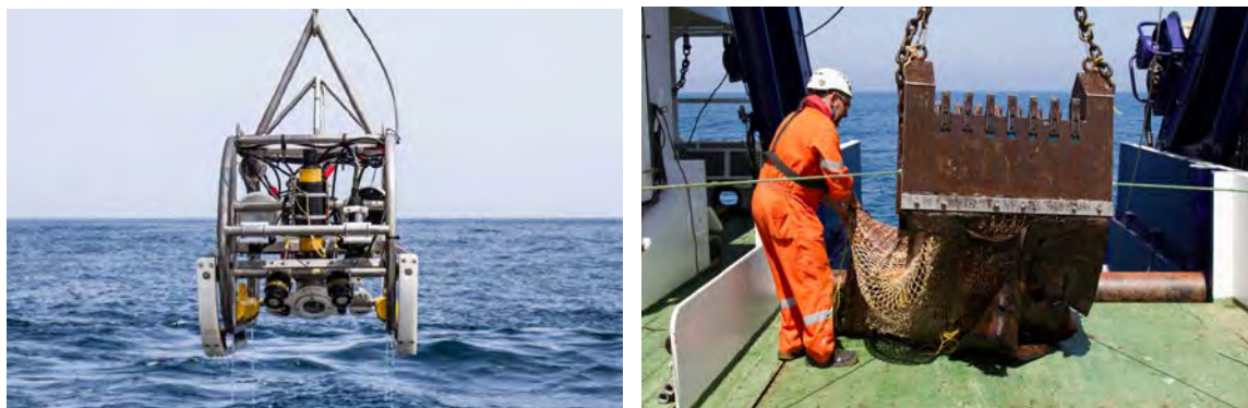
Foto 2. Muestreadores utilizados en la primera parte de la campaña: Trineo fotogramétrico Politolana (izquierda) y draga de roca (derecha).
