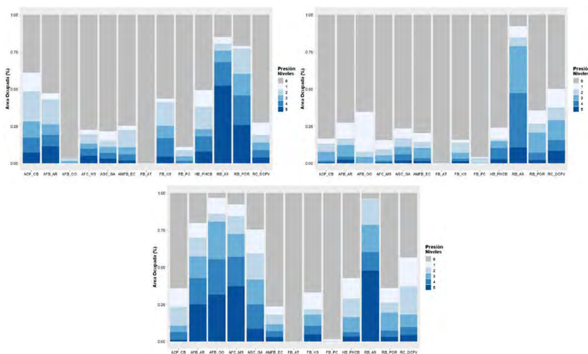
Figura 92. Área ocupada de cada hábitat bentónico por los diferentes niveles de esfuerzo pesquero palangre (izquierda), el enmalle (derecha) y arrastre (abajo). Las abreviaturas de los hábitats son: Arenas finas batiales con Actinauge richardi (AFB_AR); Arenas finas batiales con Ophiura ophiura (AFB_OO); Arenas finas circalitorales con Munida sarsi (AFC_MS); Arenas gruesas circalitorales con Gracilechinus acutus (AGC_GA); Arenas muy finas batiales con erizos de cuero (AMFB_EC); Arrecife de corales profundos ( Lophellia pertusa y Madrepora oculata ) (ACP_CB); Fangos batiales con Acanthogorgia y Thouarella (FB_AT); Fangos batiales con Kophobelemnion stelliferum (FB_KS); Fangos batiales con Pheronema carpenteri (FB_PC); Fondos de Phelliactis hertwigii con corales (HB_PHCB); Roca batial con agregaciones de esponjas (RB_POR); Roca batial con grandes esponjas hexactinellidas ( Asconema setubalense ) (RB_AS); Roca circalitoral con Dendrophyllia cornigera y Phakellia ventilabrum (RC_DCPV).
