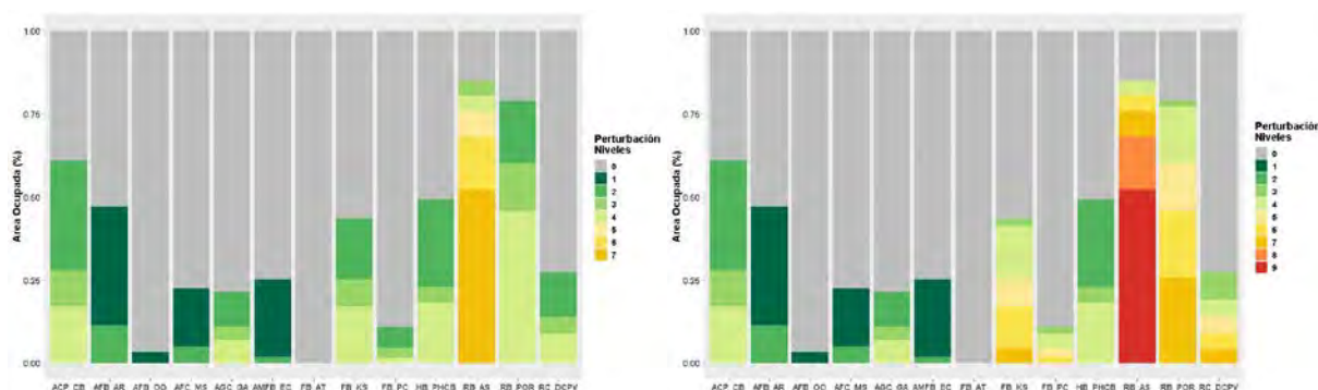
Figura 96. Área ocupada por hábitat por cada nivel de perturbación por el arte de pesca de palangre con 3 niveles (arriba) y 4 niveles (abajo) de sensibilidad. Las abreviaturas de los hábitats son: Arenas finas batiales con Actinauge richardi (AFB_AR); Arenas finas batiales con Ophiura ophiura (AFB_OO); Arenas finas circalitorales con Munida sarsi (AFC_MS); Arenas gruesas circalitorales con Gracilechinus acutus (AGC_GA); Arenas muy finas batiales con erizos de cuero (AMFB_EC); Arrecife de corales profundos ( Lophellia pertusa y Madrepora oculata ) (ACP_CB); Fangos batiales con Acanthogorgia y Thouarella (FB_AT); Fangos batiales con Kophobelemnion stelliferum (FB_KS); Fangos batiales con Pheronema carpenteri (FB_PC); Fondos de Phelliactis hertwigii con corales (HB_PHCB); Roca batial con agregaciones de esponjas (RB_POR); Roca batial con grandes esponjas hexactinellidas ( Asconema setubalense ) (RB_AS); Roca circalitoral con Dendrophyllia cornigera y Phakellia ventilabrum (RC_DCPV).
